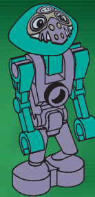
MIZAR
