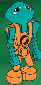
VEGA
