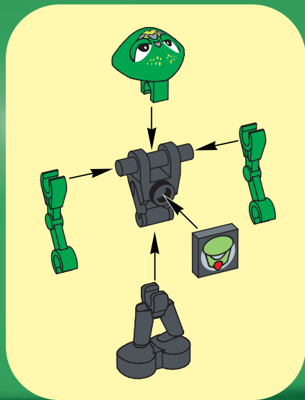
RIGEL
